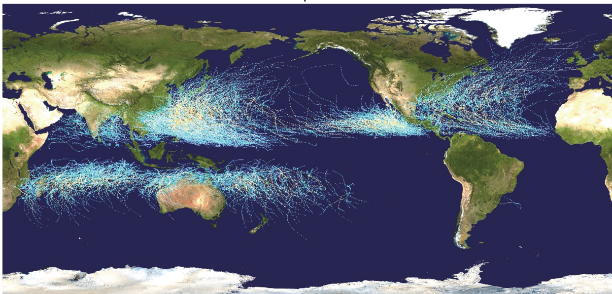
Mapa 1.
