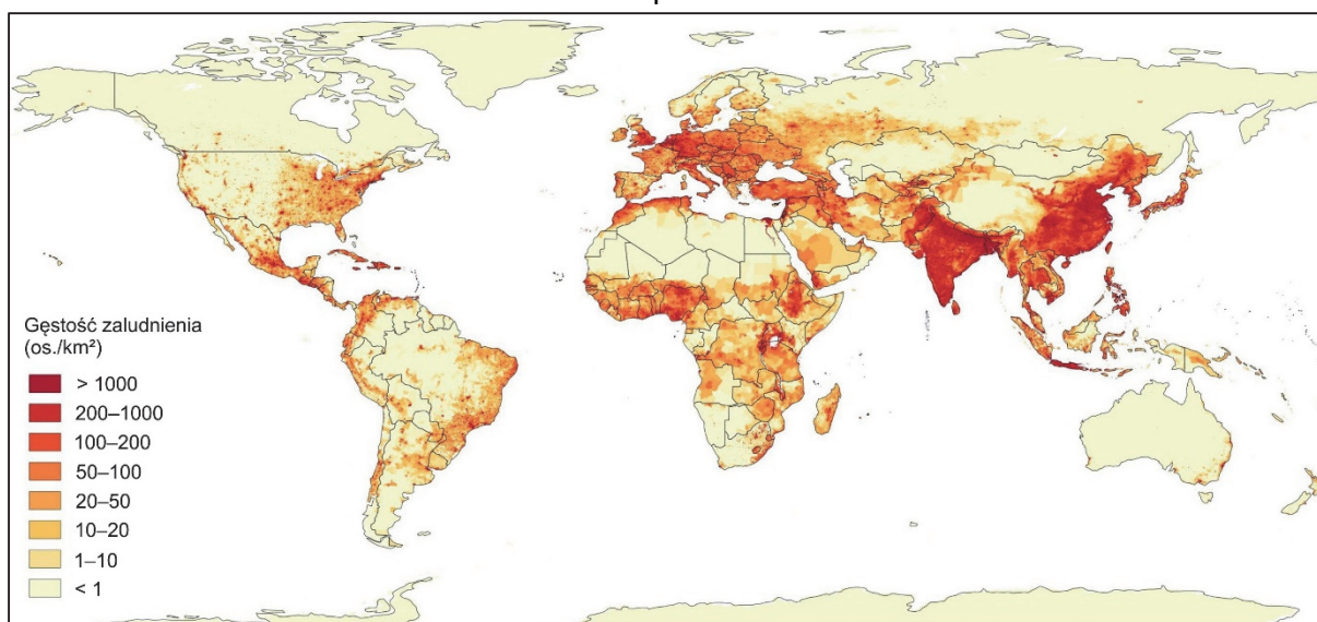
Mapa 2.
