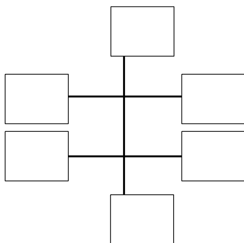
erytrol
