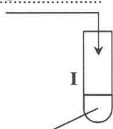
cykloheksan
